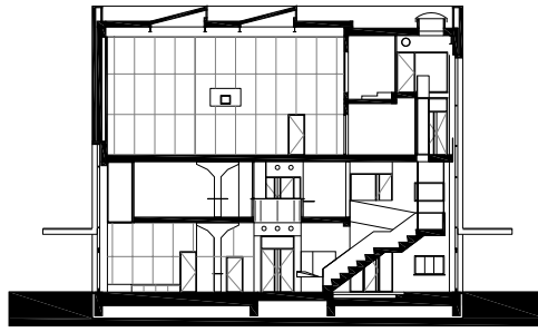
Doorsnede A-A
