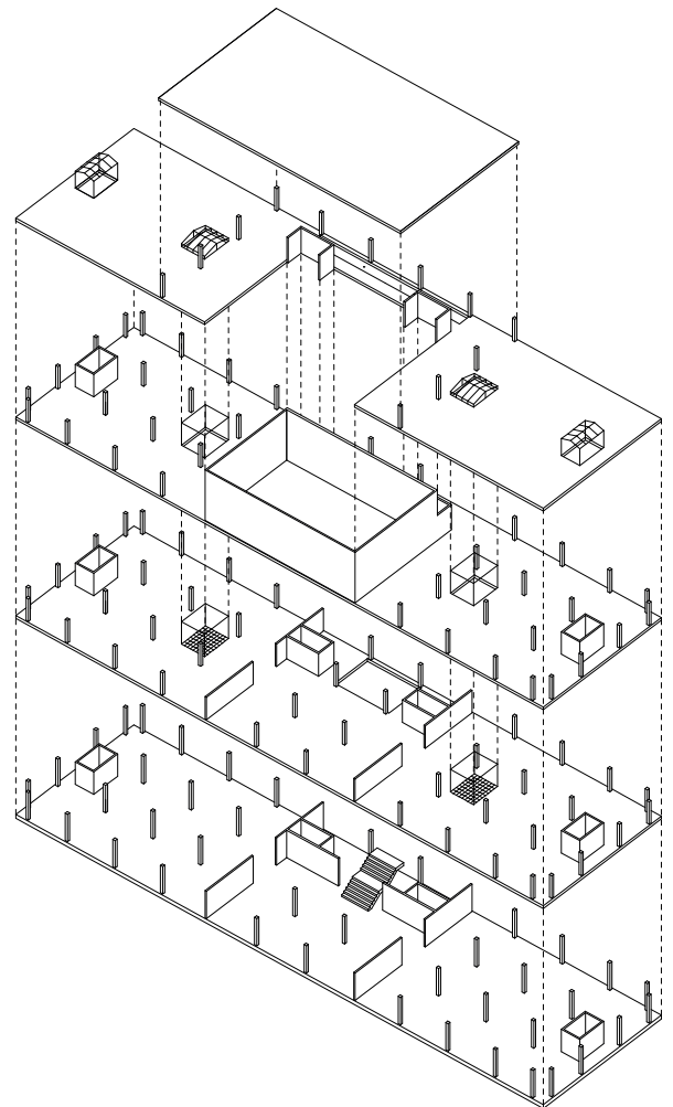
FLEXIBEL GEBOUW MET GENERIEKE HOOFDDRAAGCONSTRUCTIE
