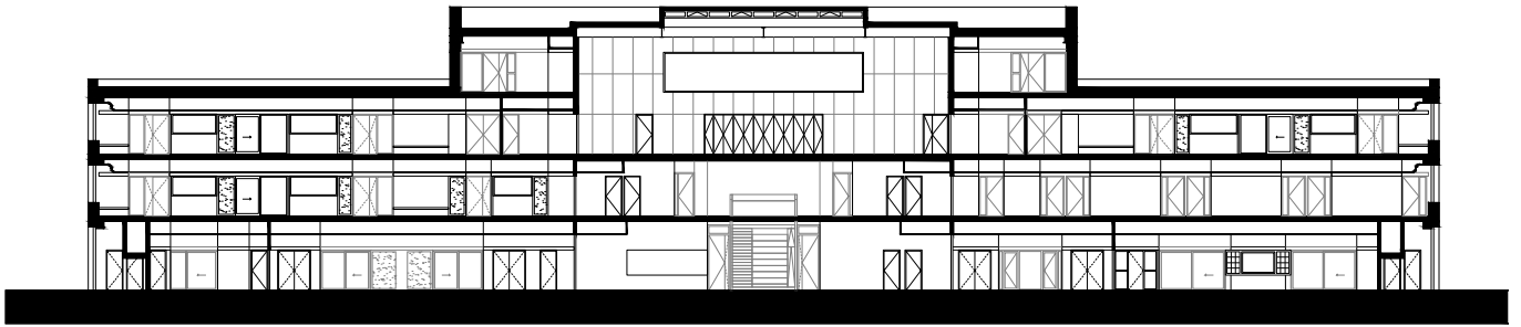
Doorsnede B-B
